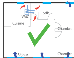
→ Air neuf → Air vicié → Défauts d'étanchéité
