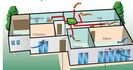
Bouches d'extraction hygro réglables Entrées d'air hygro réglables → Air neuf → Air vicié ■ Groupe d'extraction
